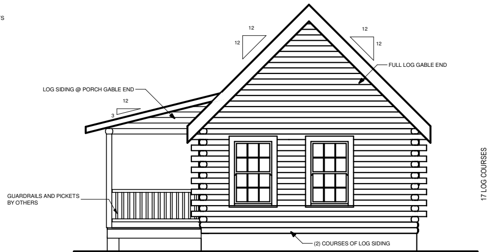
RIGHT ELEVATION
