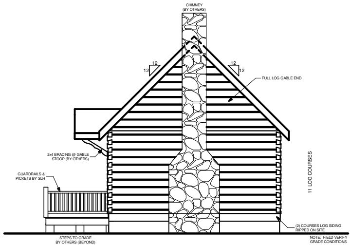
RIGHT ELEVATION
