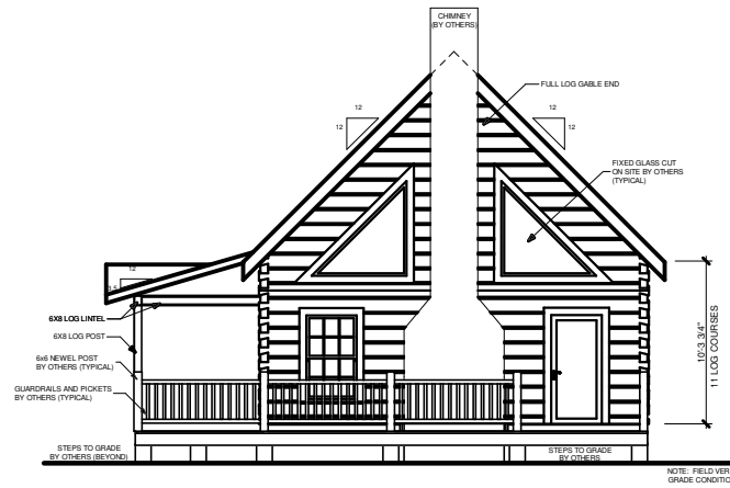
RIGHT ELEVATION 14'x11'0"
