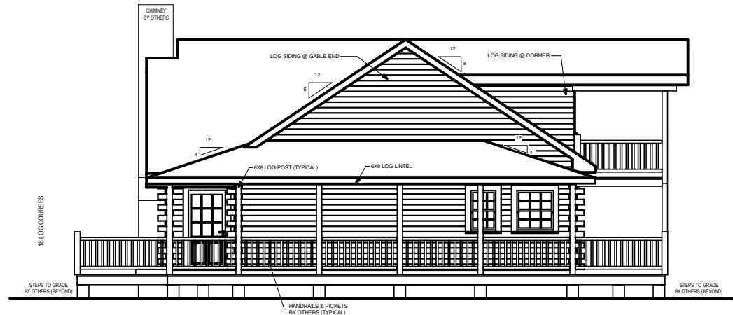
RIGHT ELEVATION
