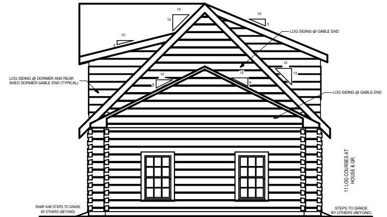
RIGHT ELEVATION
