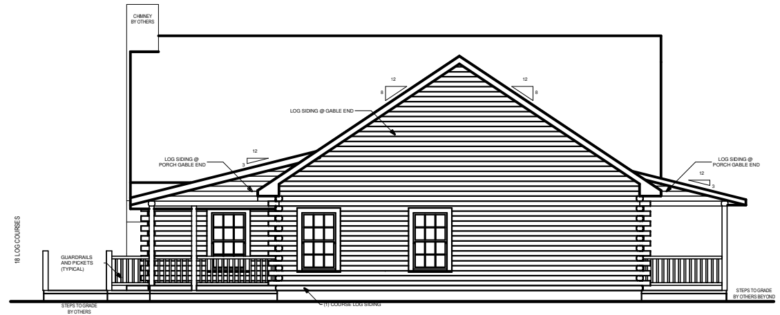
RIGHT ELEVATION
