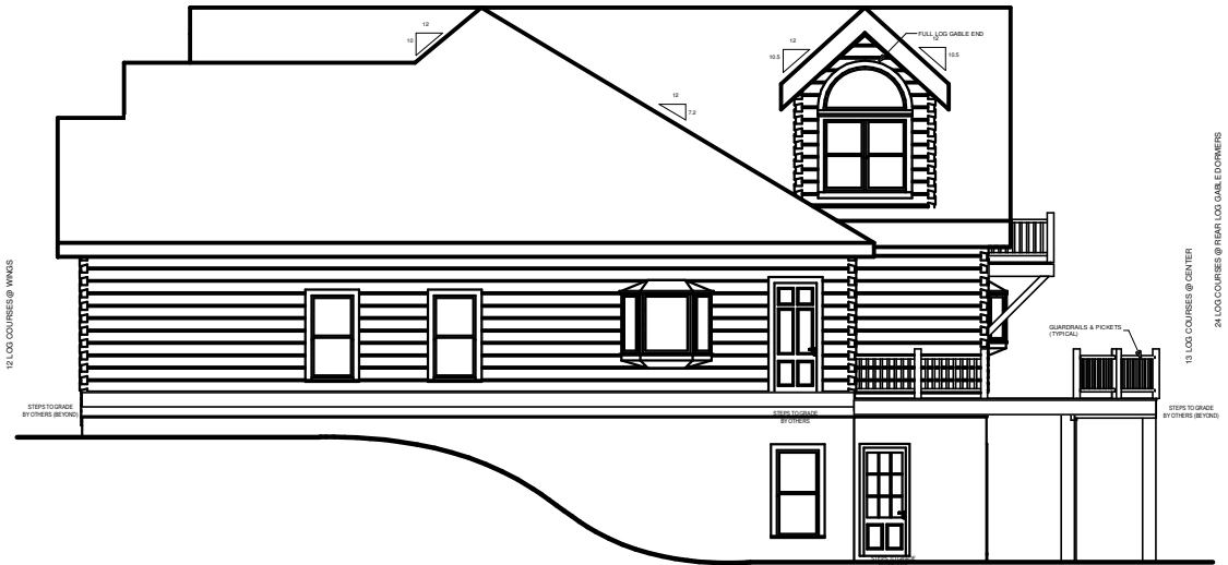
RIGHT ELEVATION
