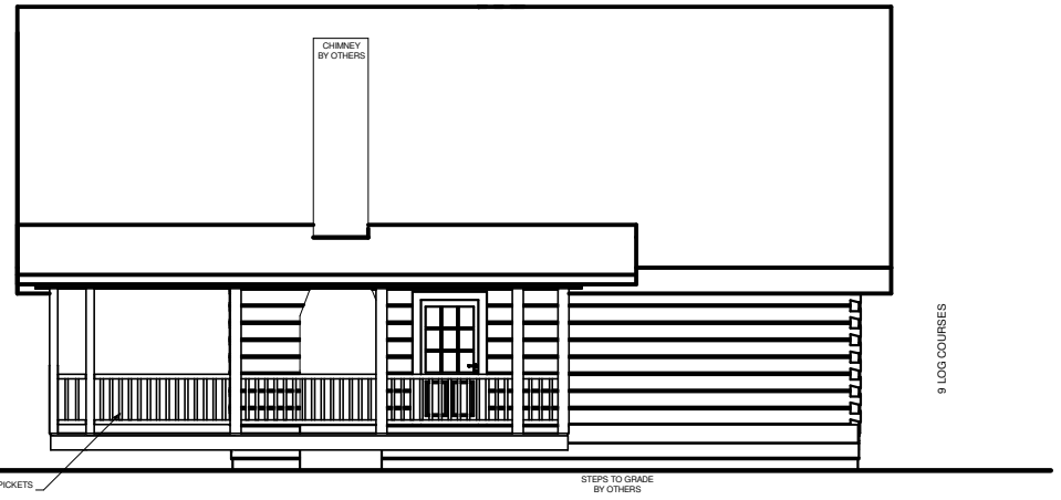
RIGHT ELEVATION
