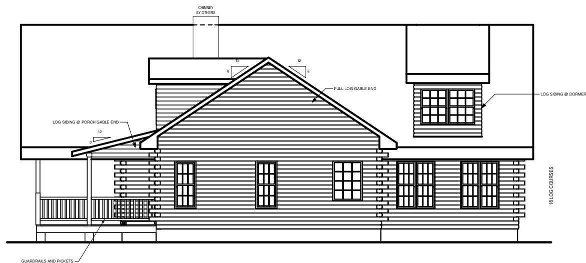
RIGHT ELEVATION
