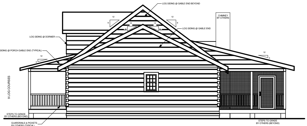
RIGHT ELEVATION
