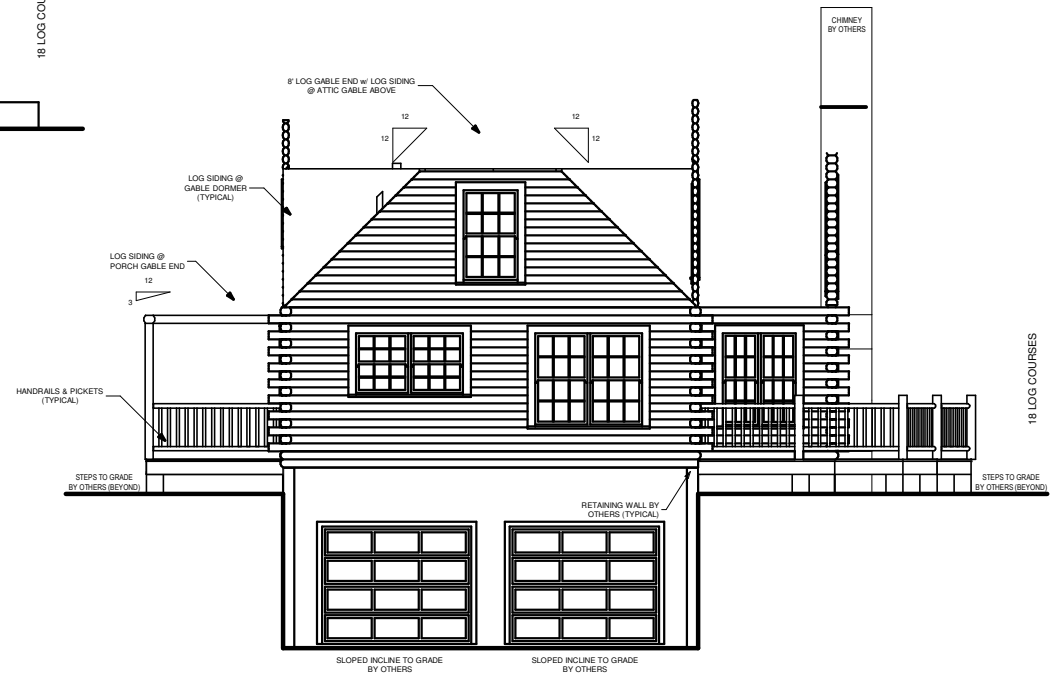
RIGHT ELEVATION
