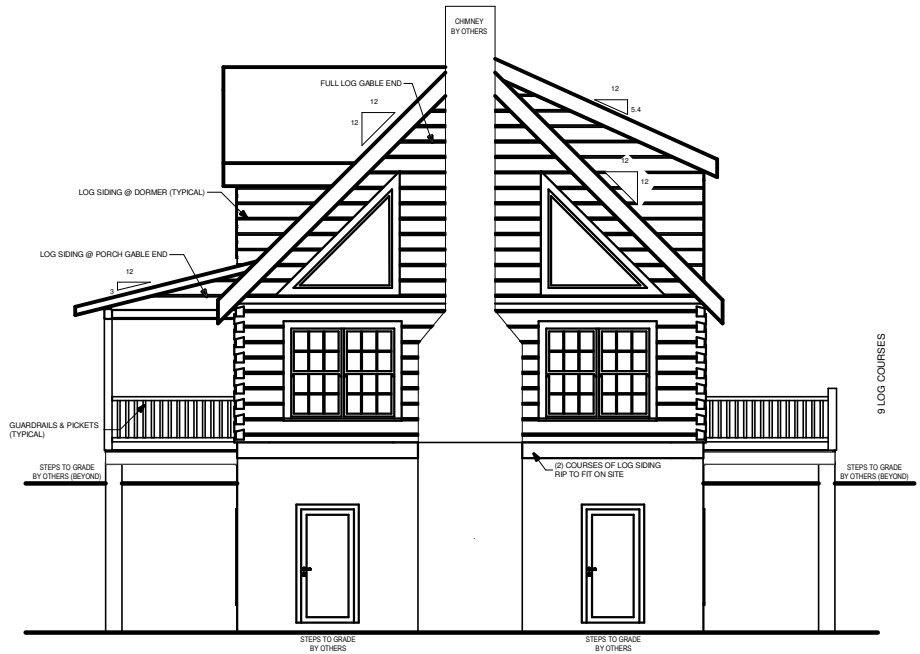
RIGHT ELEVATION
