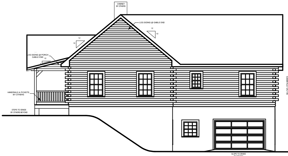
RIGHT ELEVATION
