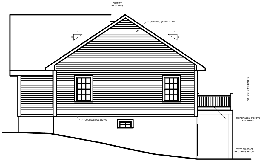
RIGHT ELEVATION
