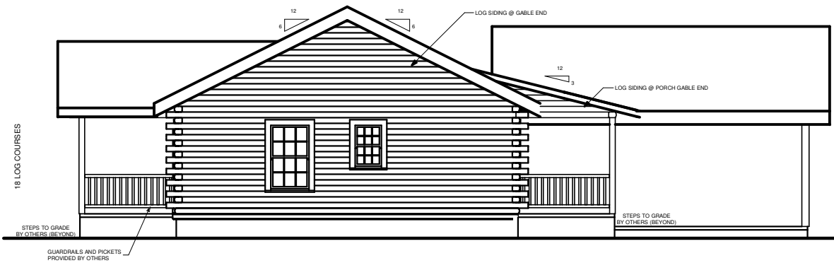
RIGHT ELEVATION
