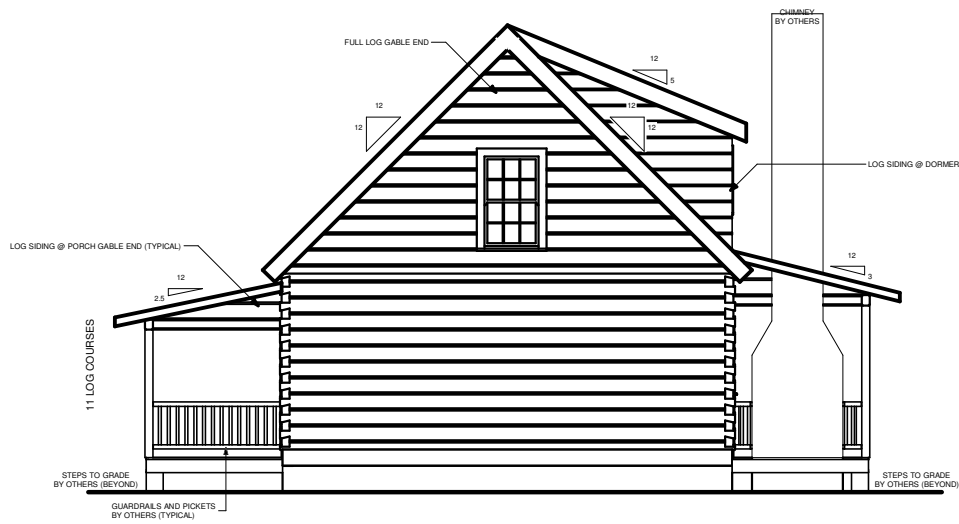
RIGHT ELEVATION
