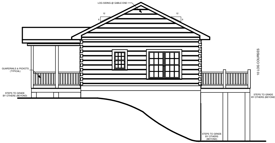
RIGHT ELEVATION
