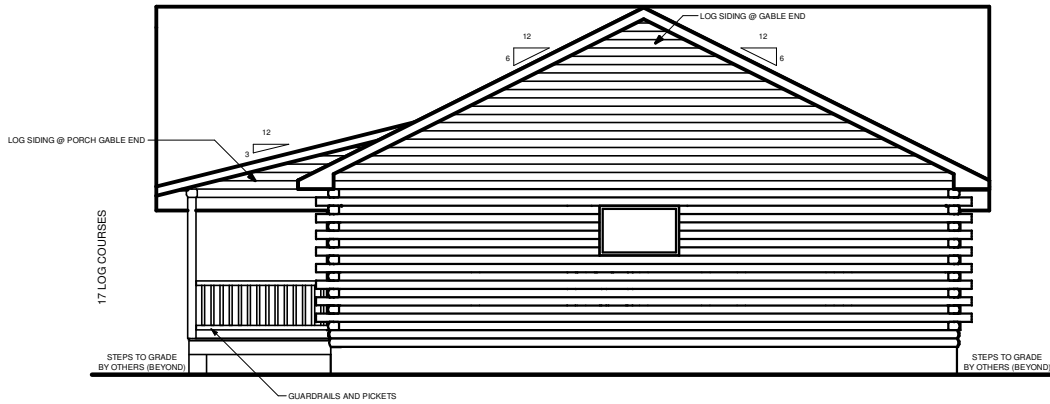
RIGHT ELEVATION
