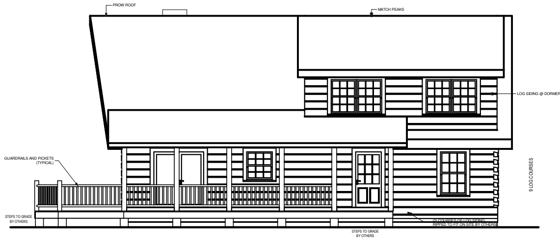
RIGHT ELEVATION
