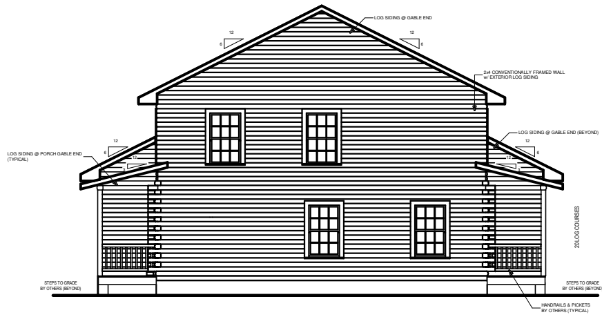
RIGHT ELEVATION
