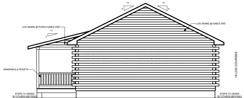
RIGHT ELEVATION
