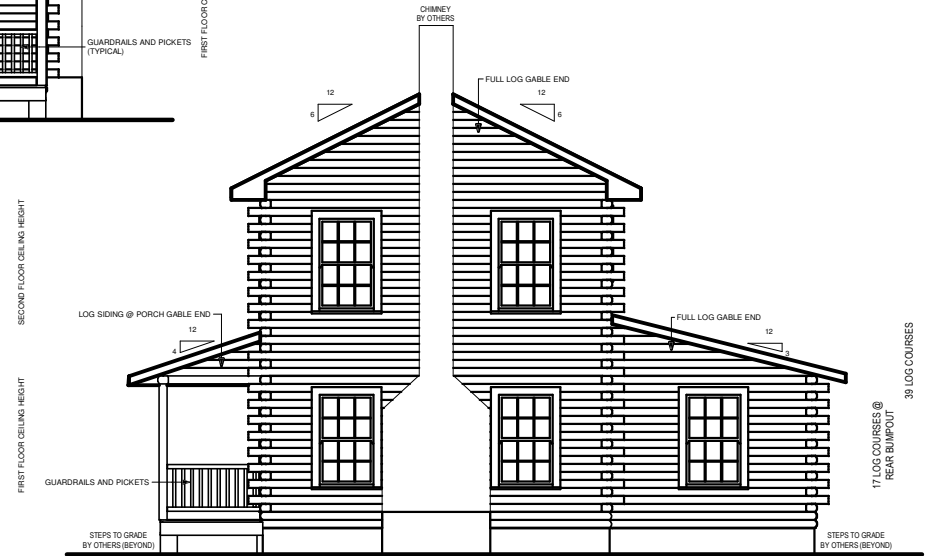
RIGHT ELEVATION
