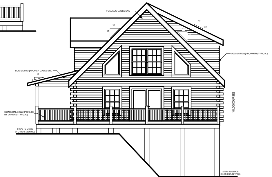
RIGHT ELEVATION
