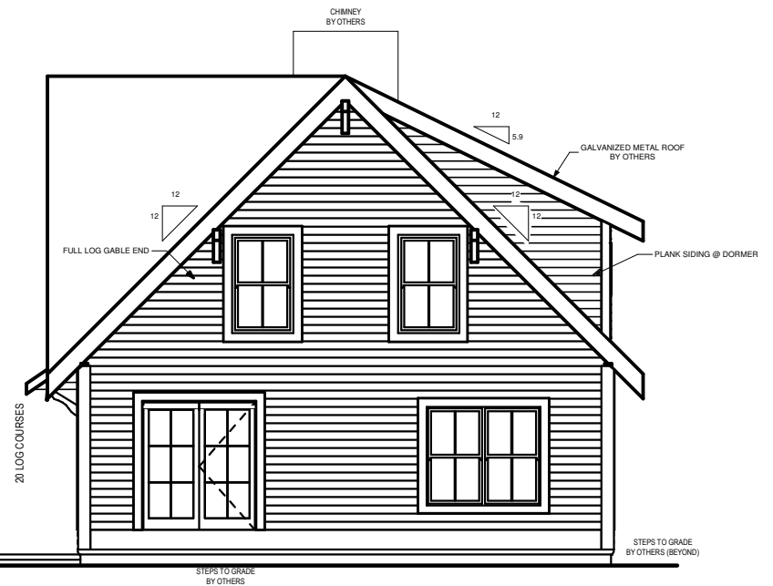
RIGHT ELEVATION
