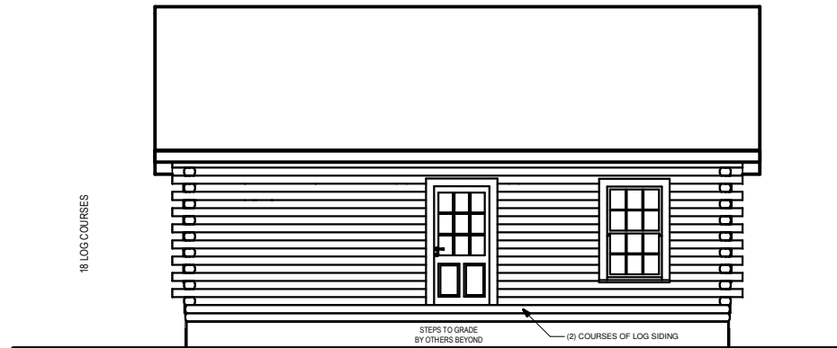
RIGHT ELEVATION
